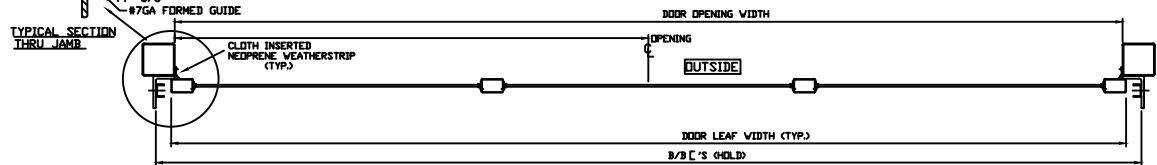
SECTION A-A
